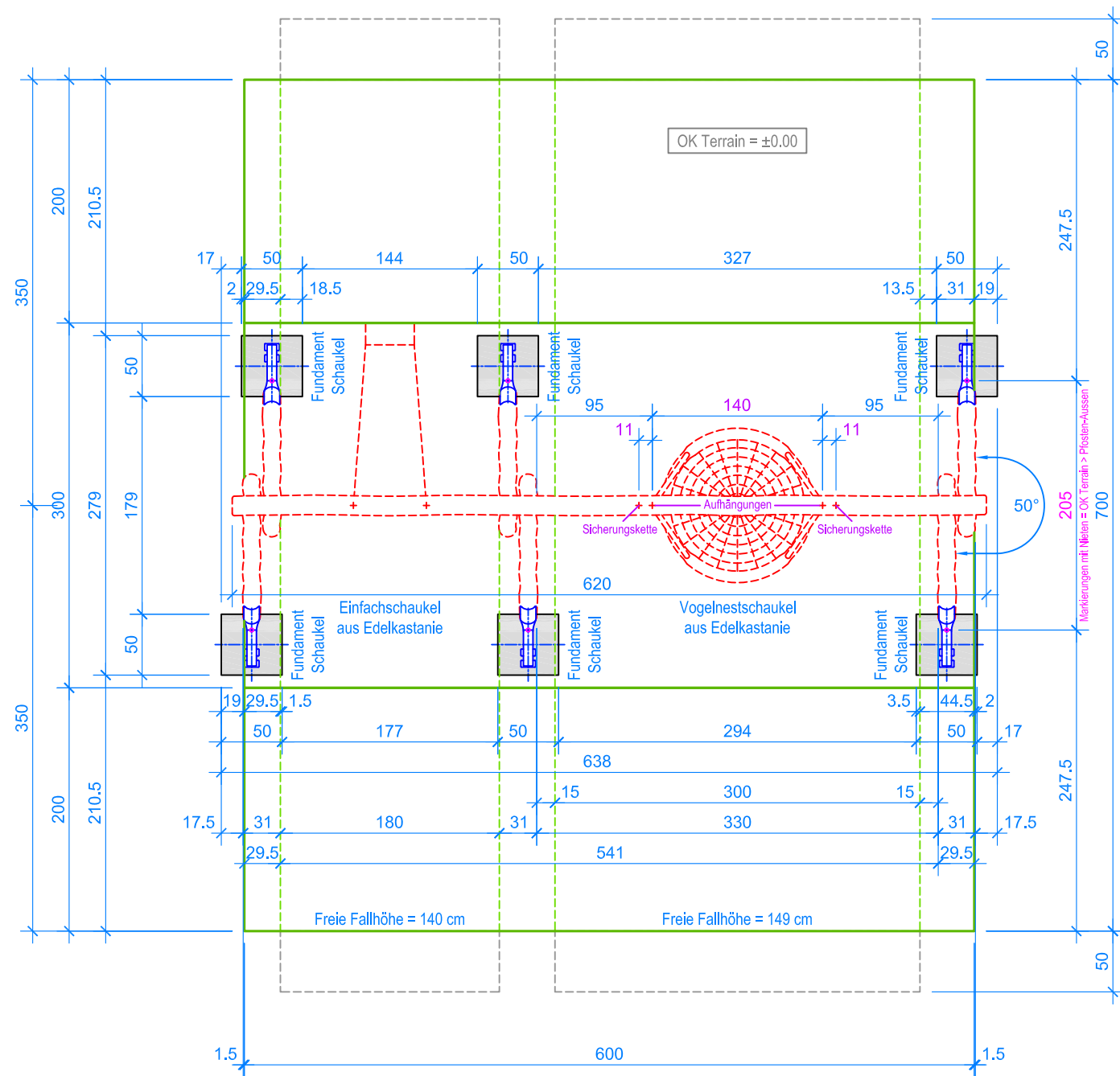
GRUNDRISS 1:50
