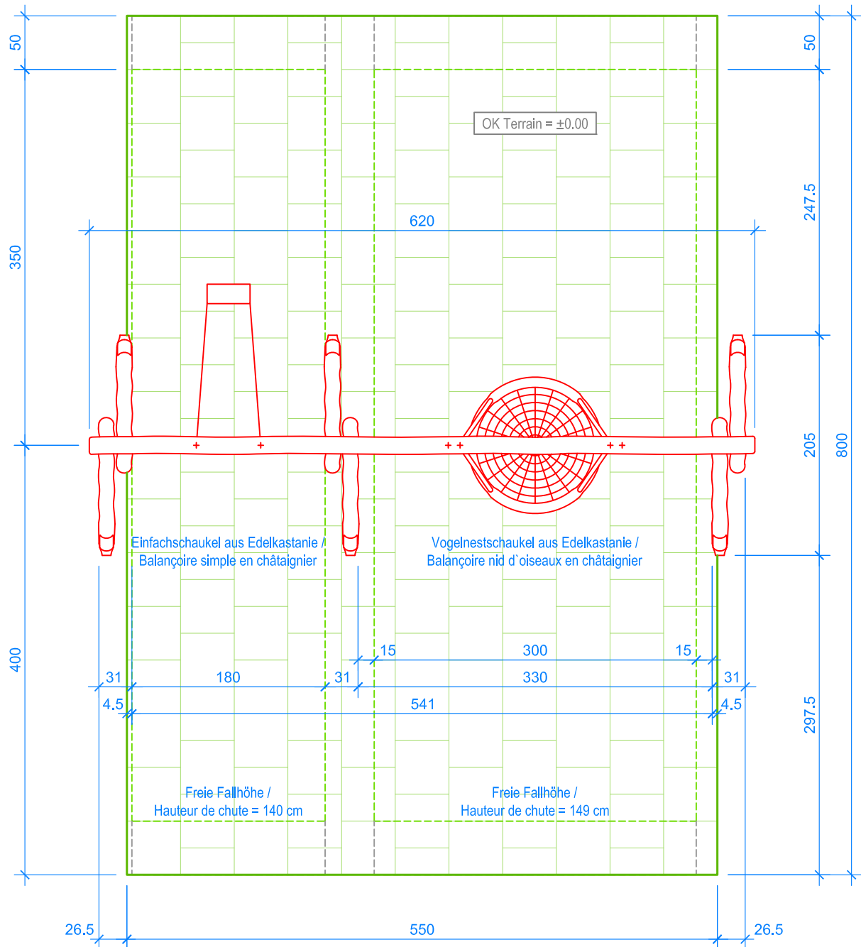
GRUNDRISS / PLAN 1:50
