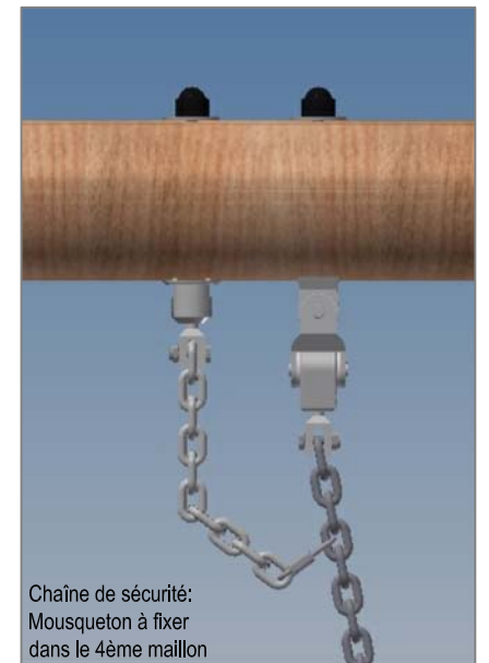
Détail A
