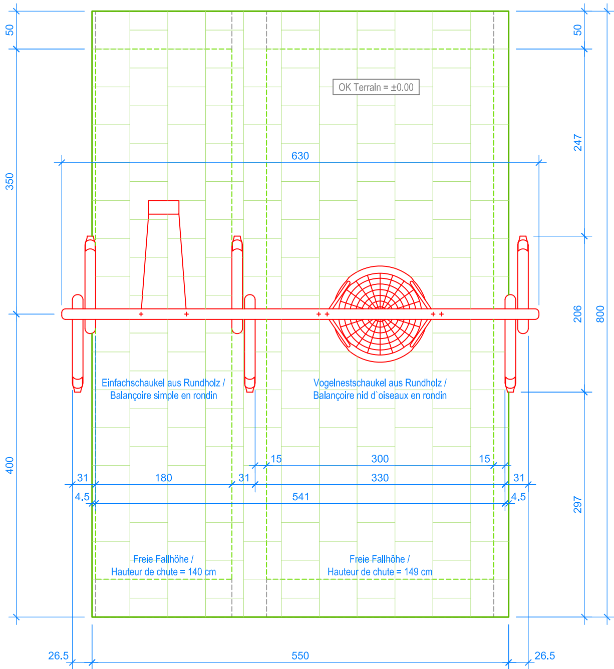
GRUNDRISS / PLAN 1:50
