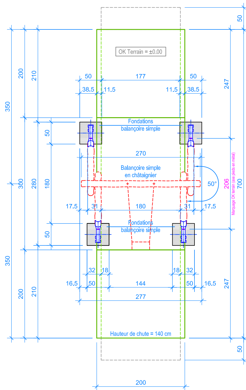
PLAN 1:50
