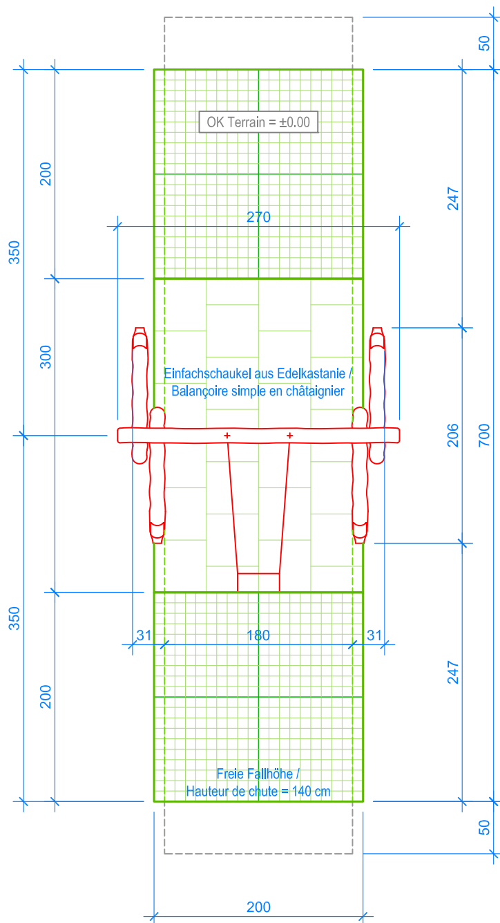
GRUNDRISS / PLAN 1:50
