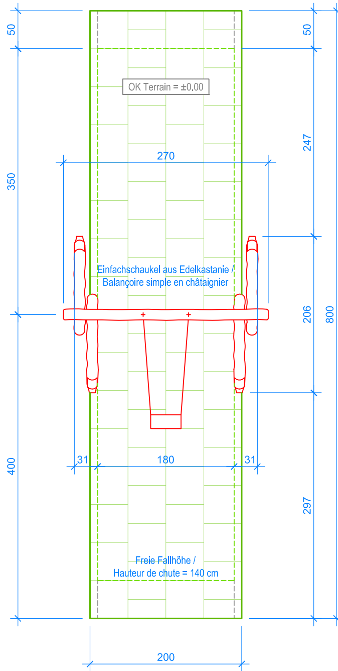
GRUNDRISS / PLAN 1:50
