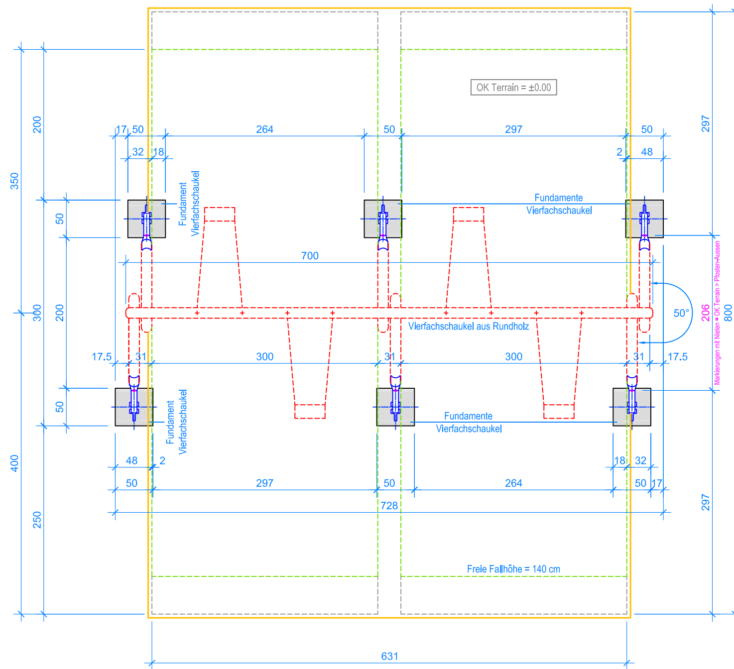
GRUNDRISS 1:50
