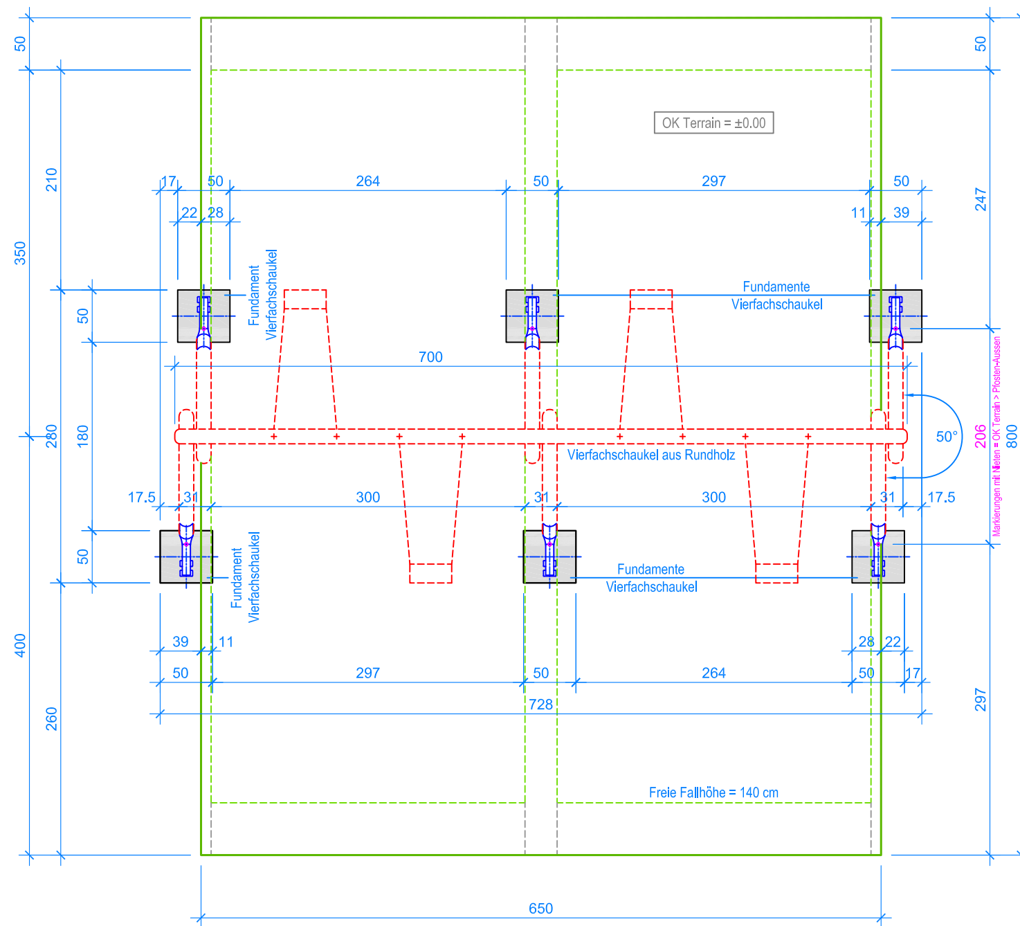
GRUNDRISS 1:50
