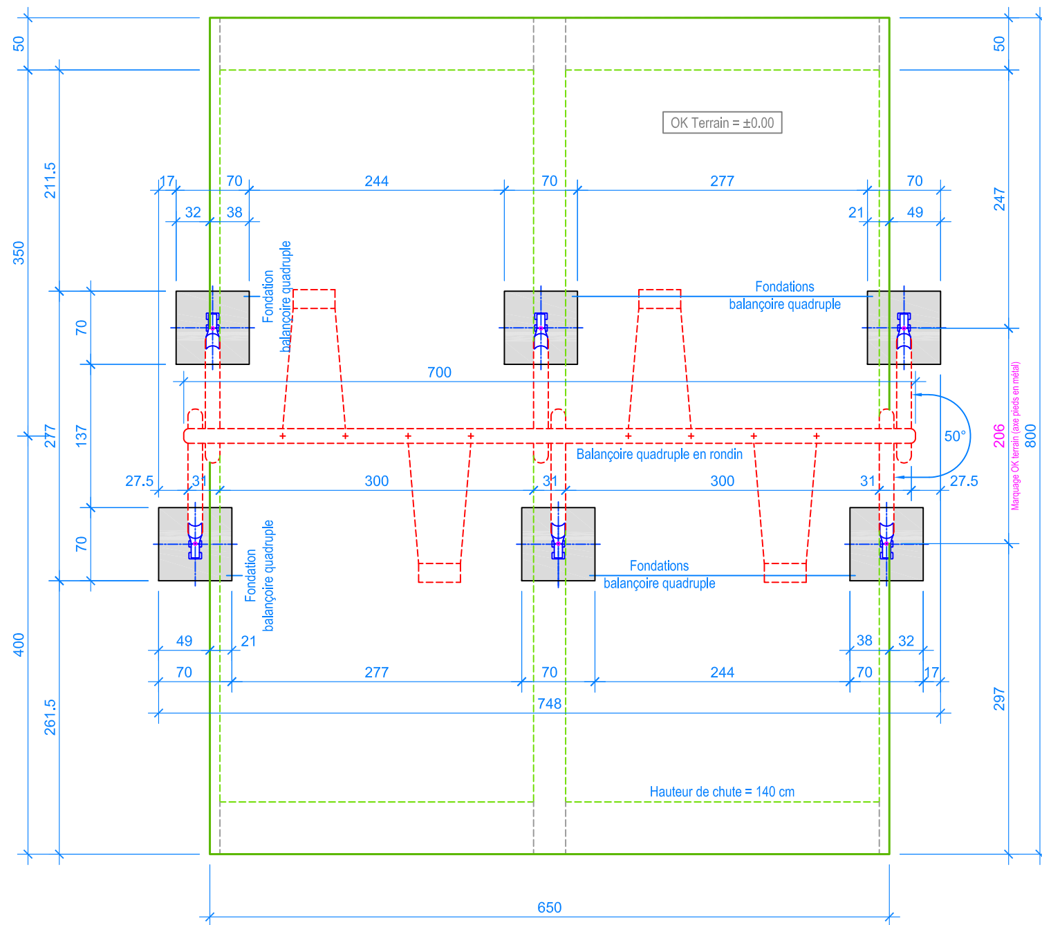
PLAN 1:50
