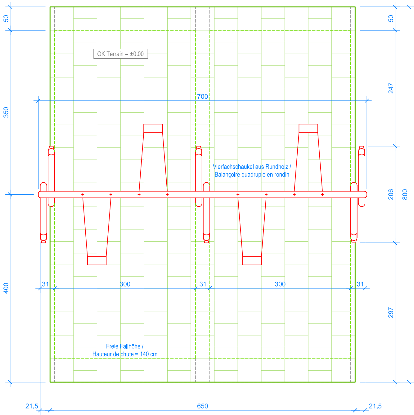
GRUNDRISS / PLAN 1:50
