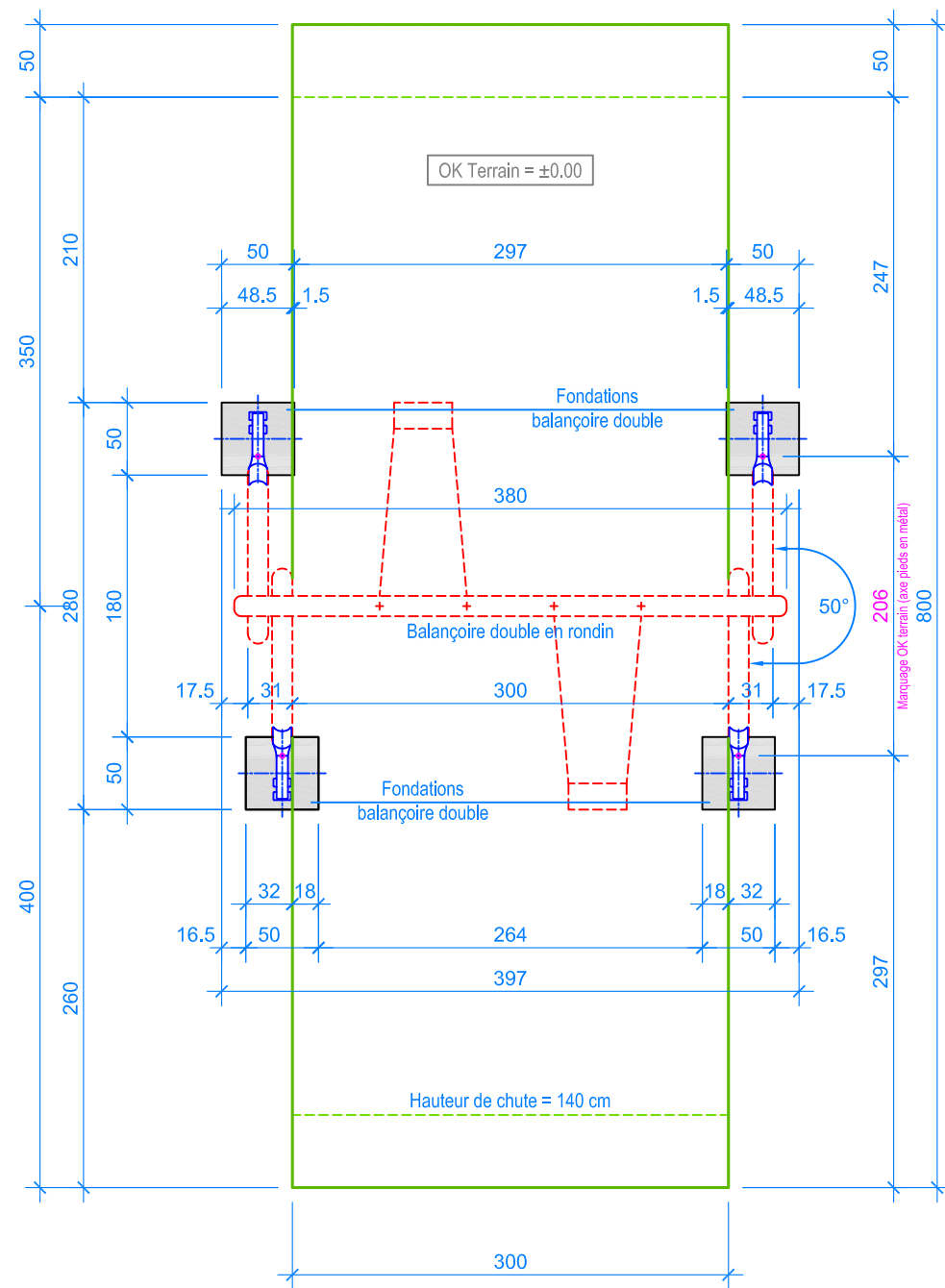
PLAN 1:50
