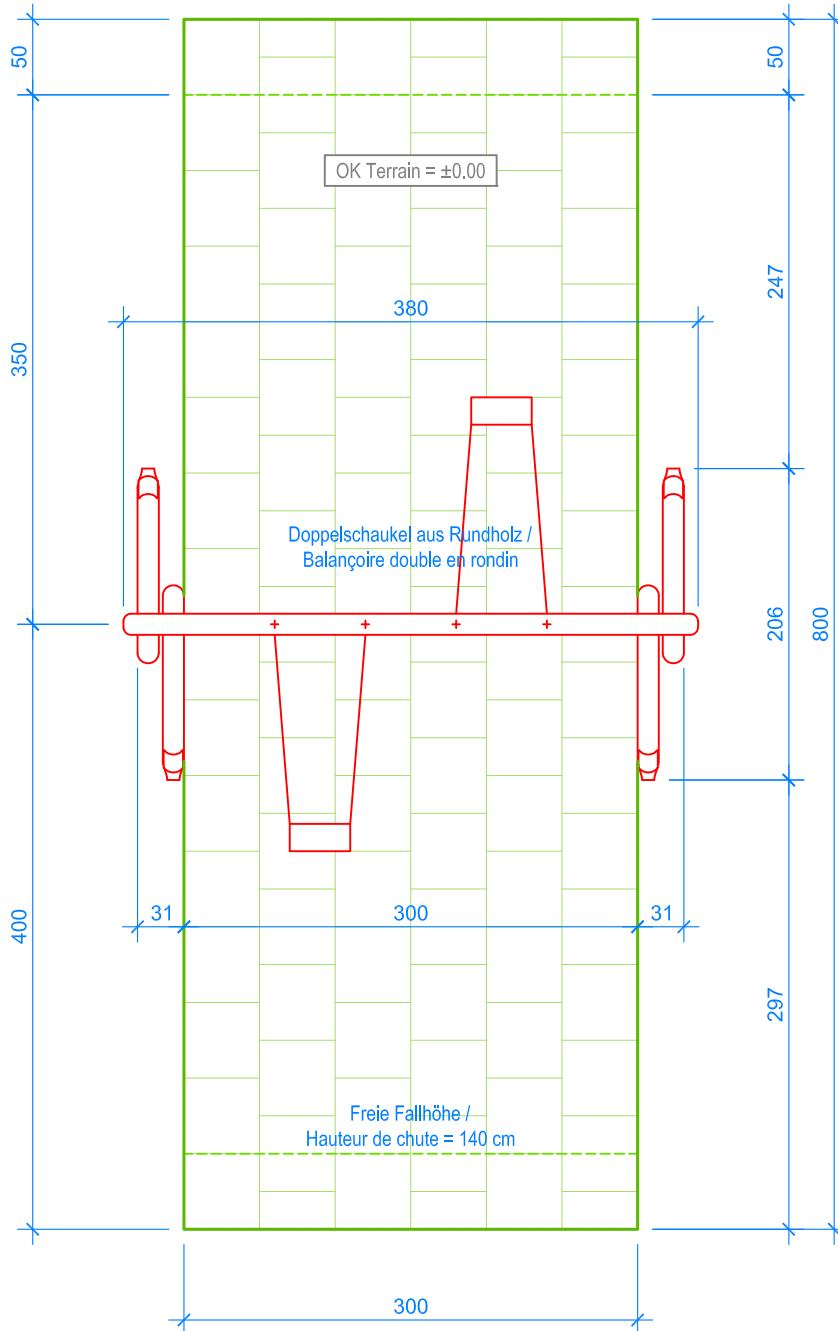
GRUNDRISS / PLAN 1:50
