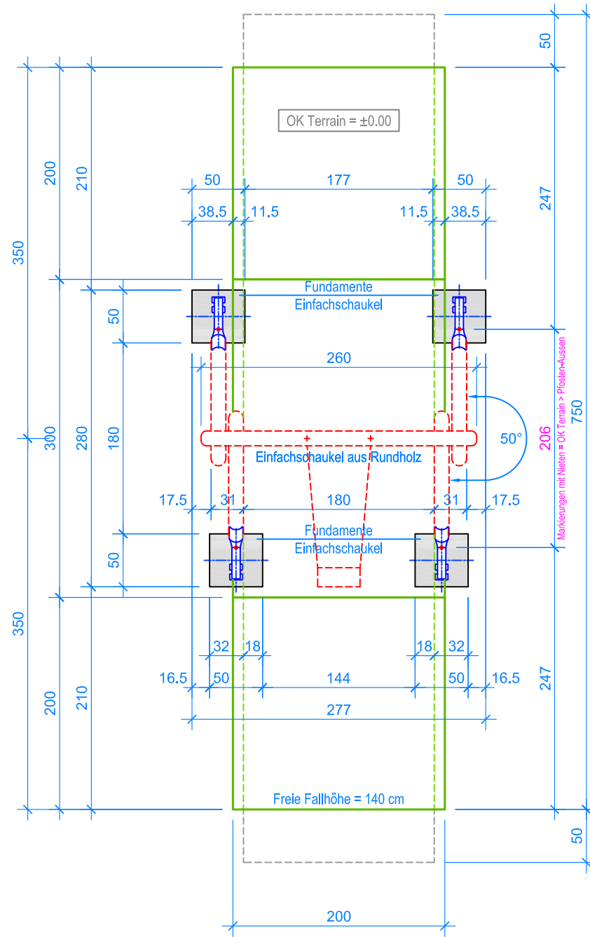
GRUNDRISS 1:50
