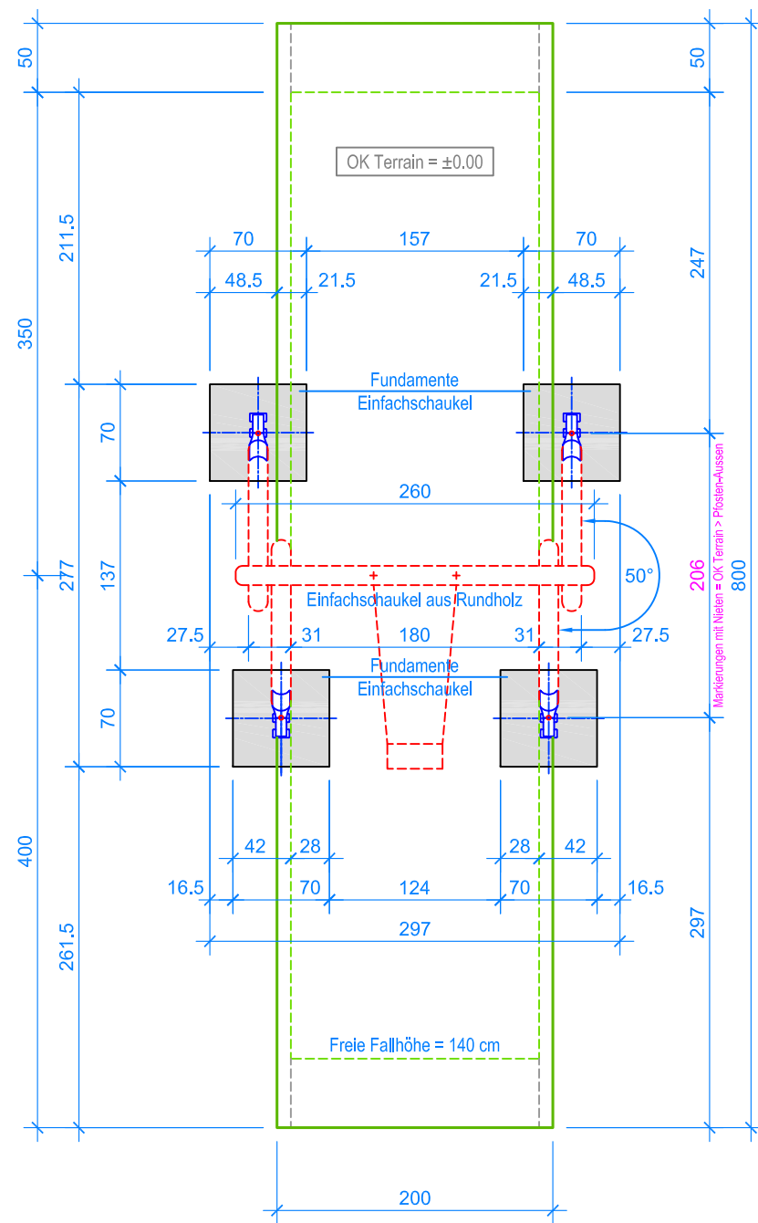
GRUNDRISS 1:50
