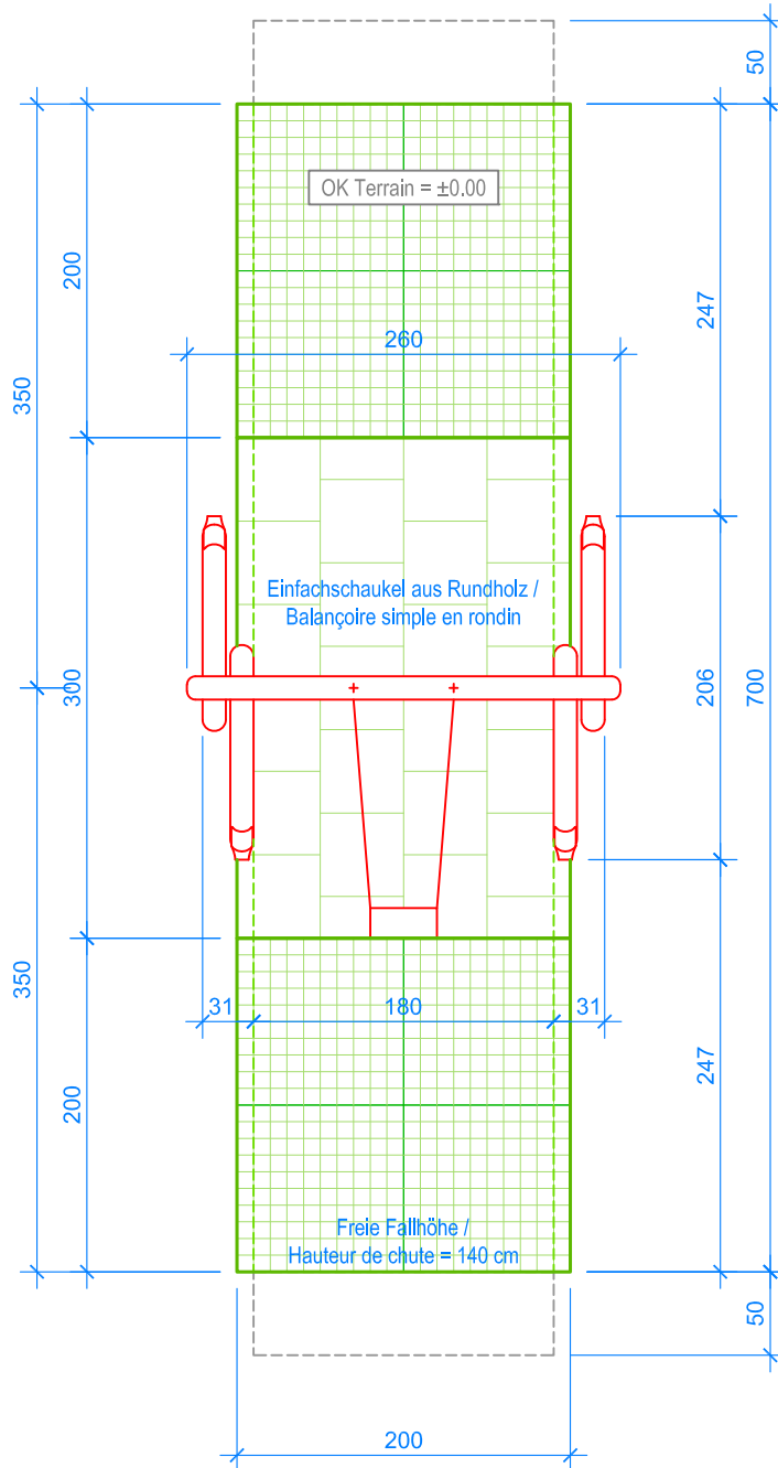
GRUNDRISS / PLAN 1:50
