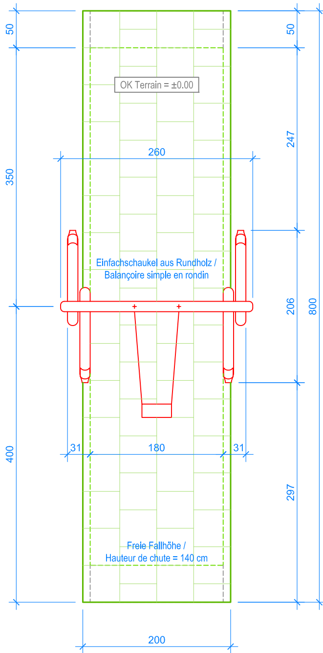
GRUNDRISS / PLAN 1:50
