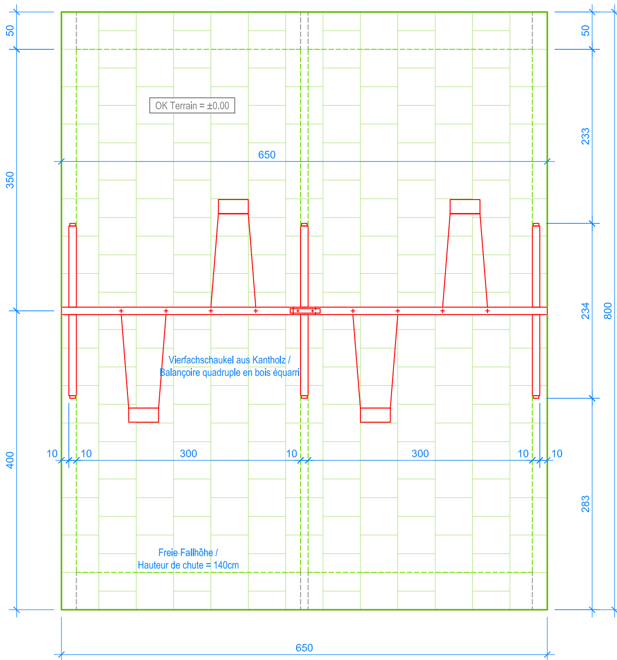
GRUNDRISS / PLAN 1:50
