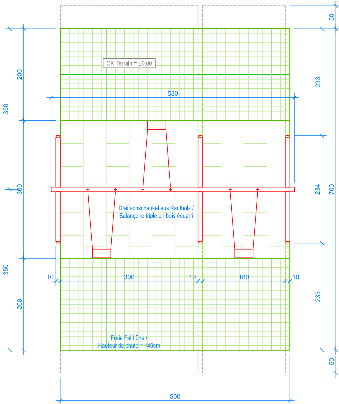
GRUNDRISS / PLAN 1:50
