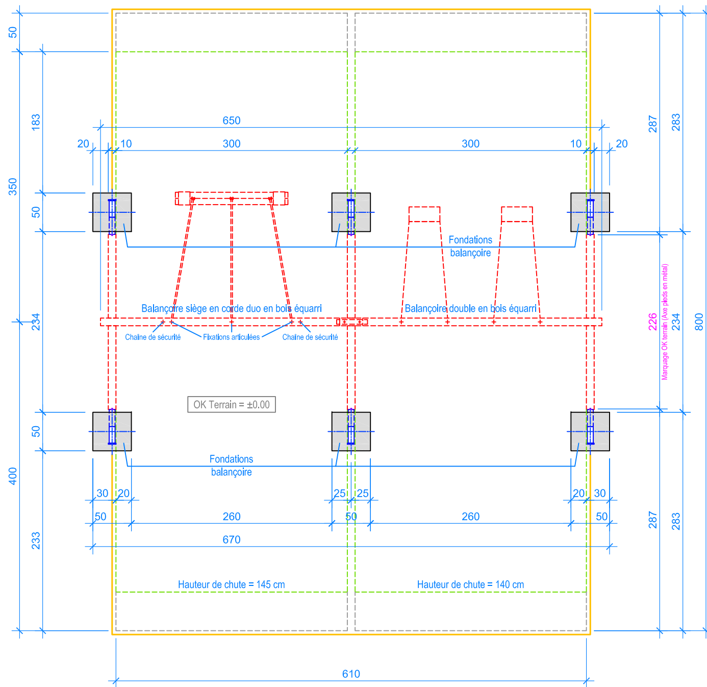
PLAN 1:50
