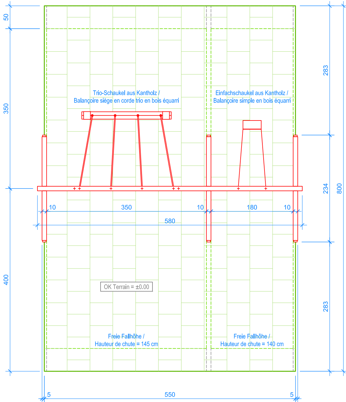
GRUNDRISS / PLAN 1:50
