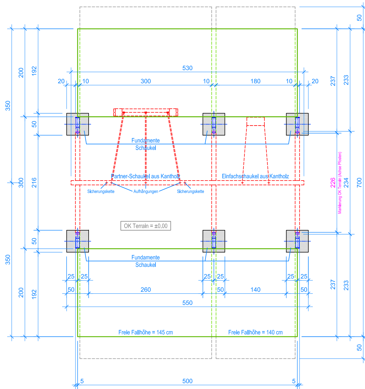
GRUNDRISS 1:50
