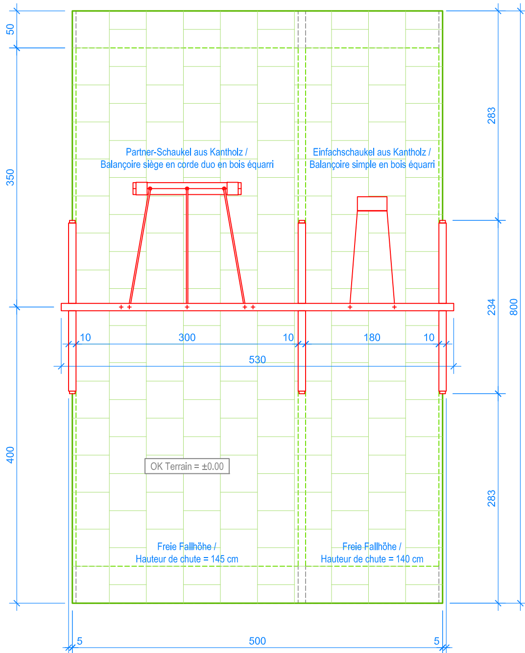
GRUNDRISS / PLAN 1:50
