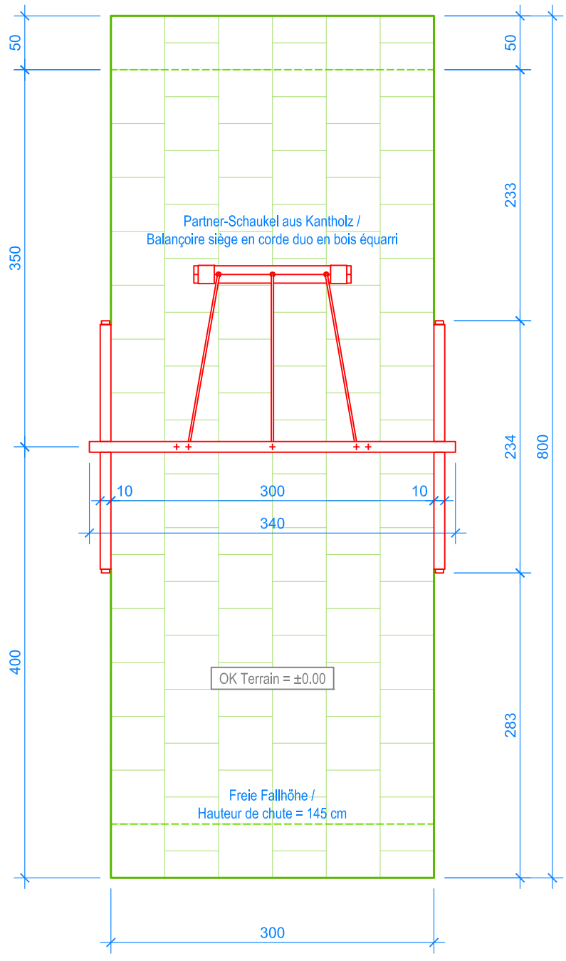
GRUNDRISS / PLAN 1:50
