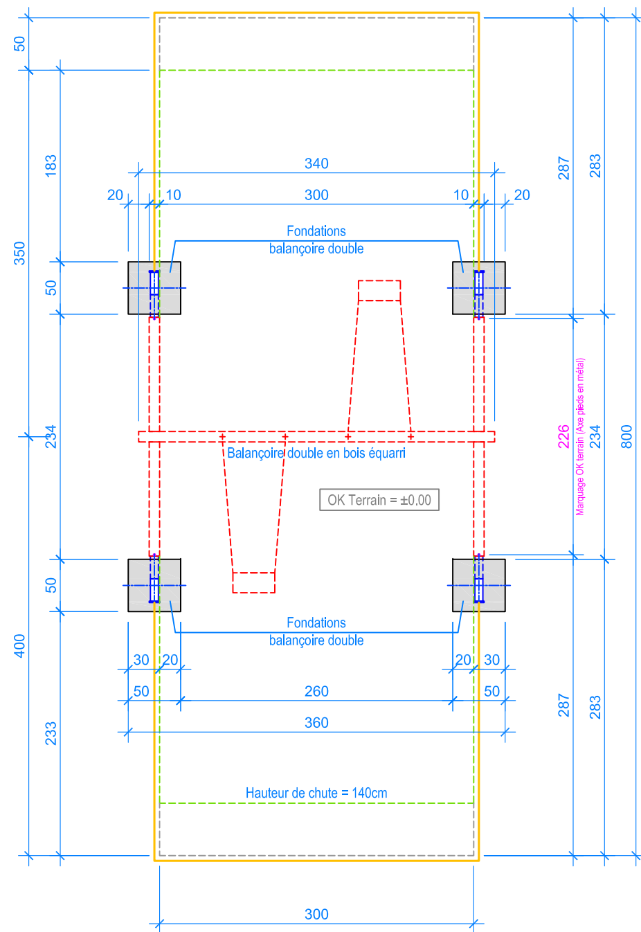
PLAN 1:50
