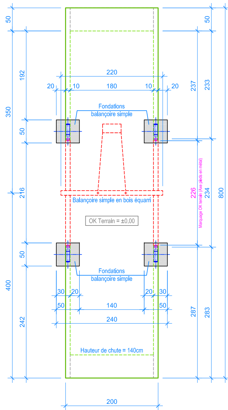
PLAN 1:50
