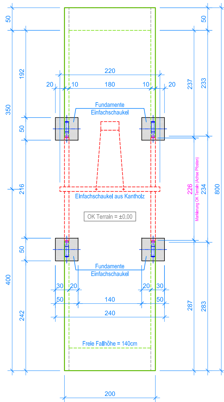
GRUNDRISS 1:50
