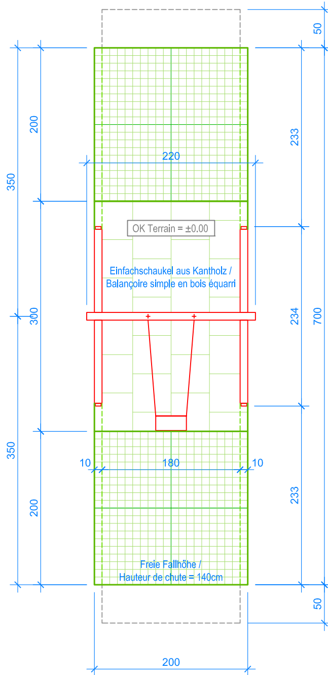
GRUNDRISS / PLAN 1:50
