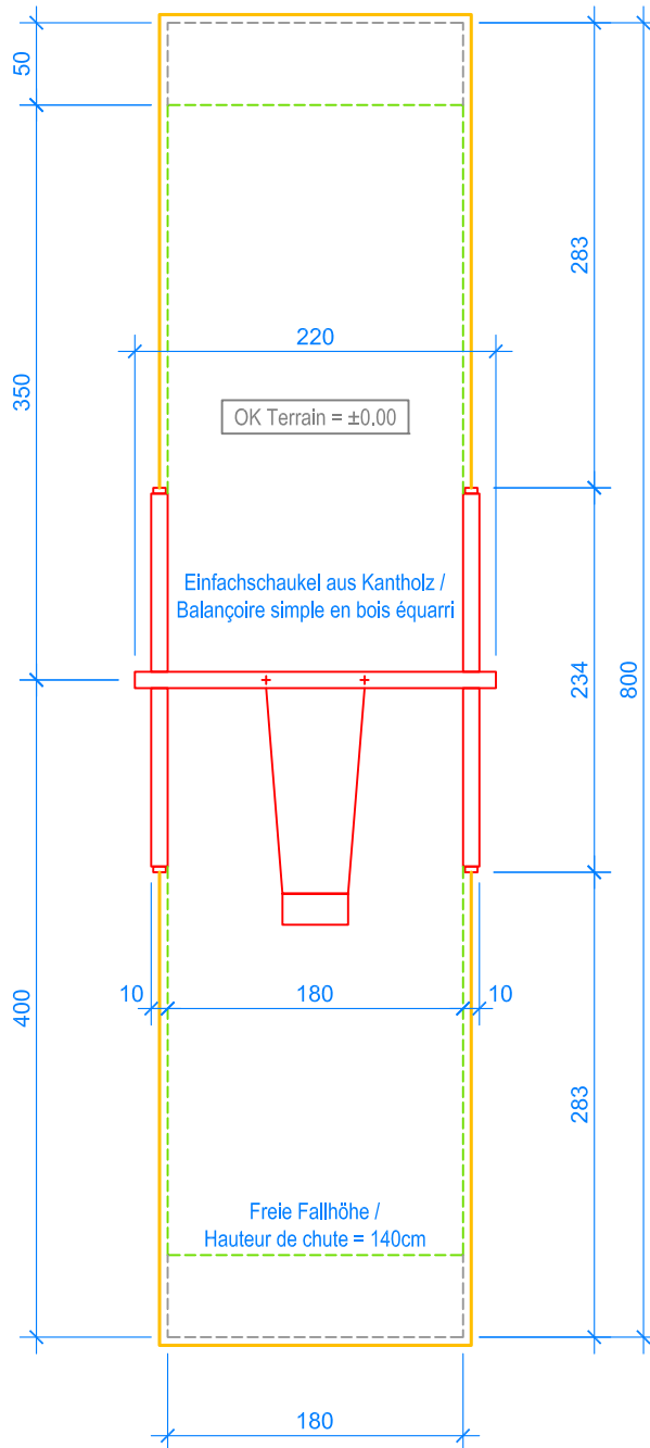
GRUNDRISS / PLAN 1:50
