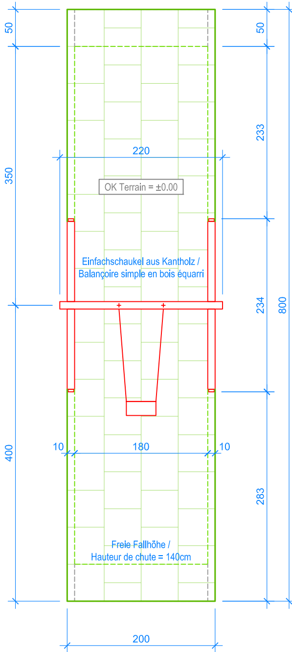
GRUNDRISS / PLAN 1:50
