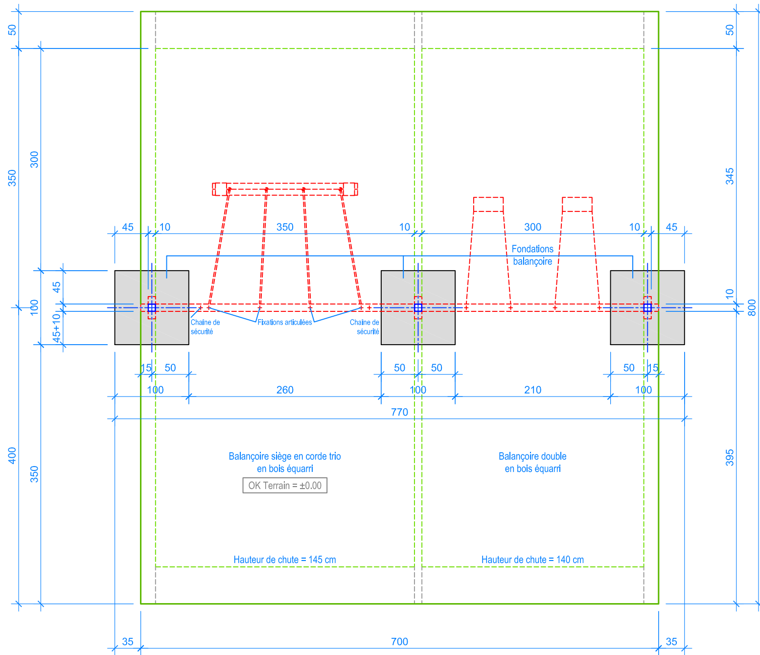
PLAN 1:50
