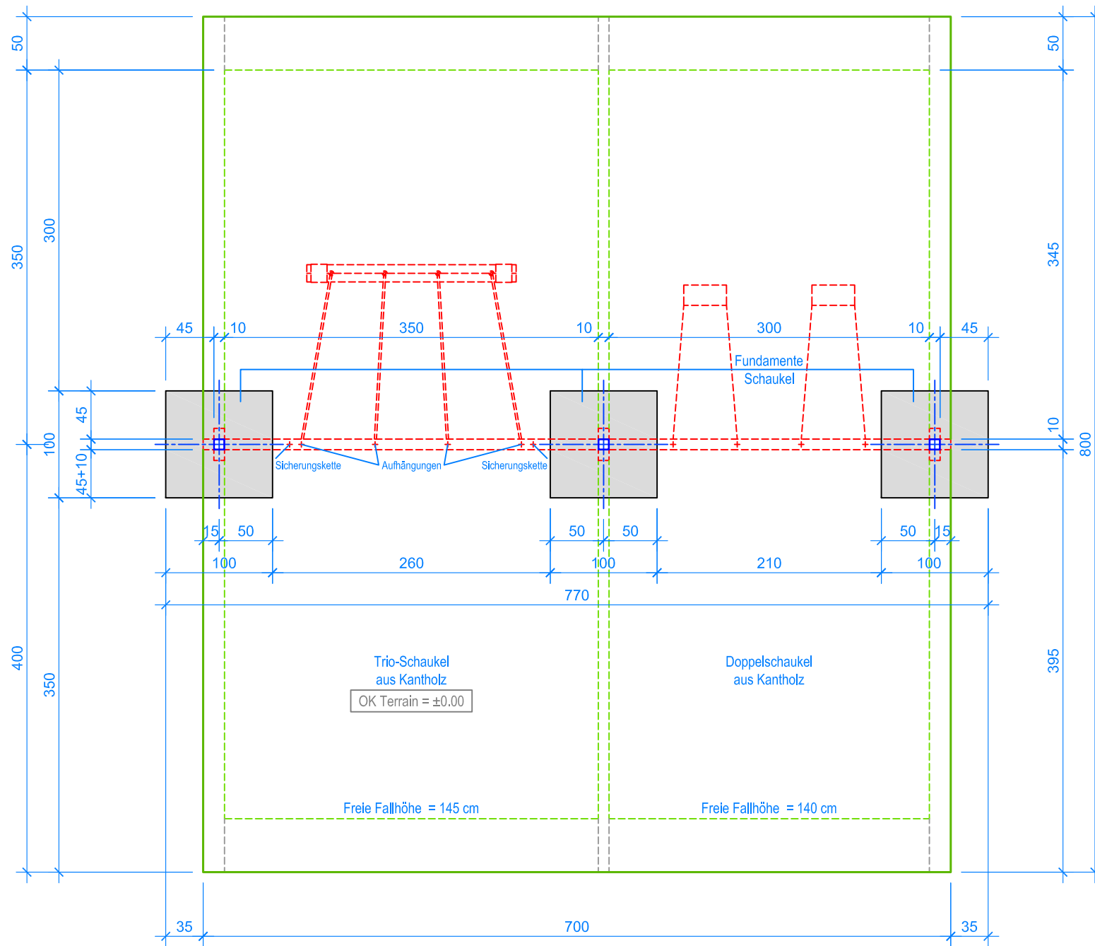
GRUNDRISS 1:50
