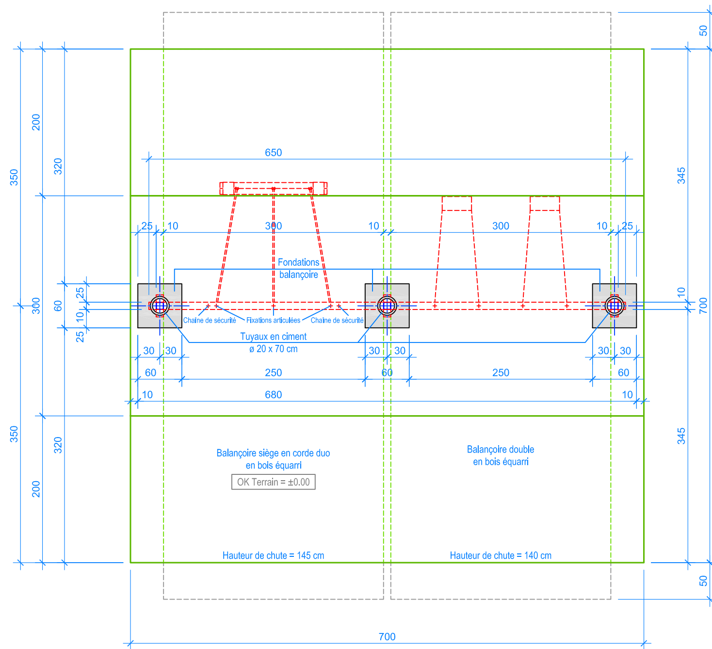
PLAN 1:50
