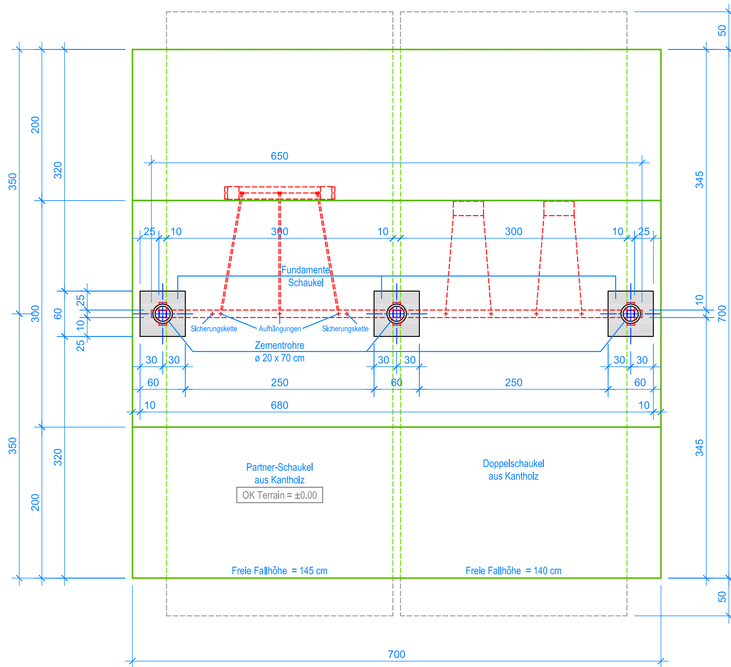
GRUNDRISS 1:50
