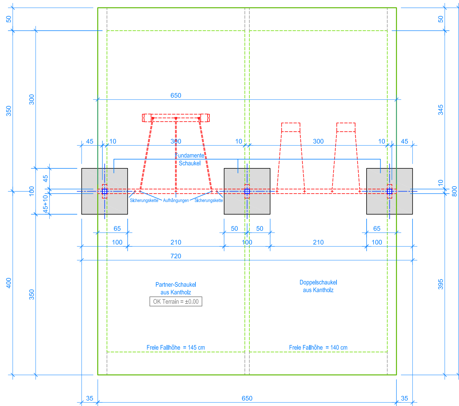
GRUNDRISS 1:50
