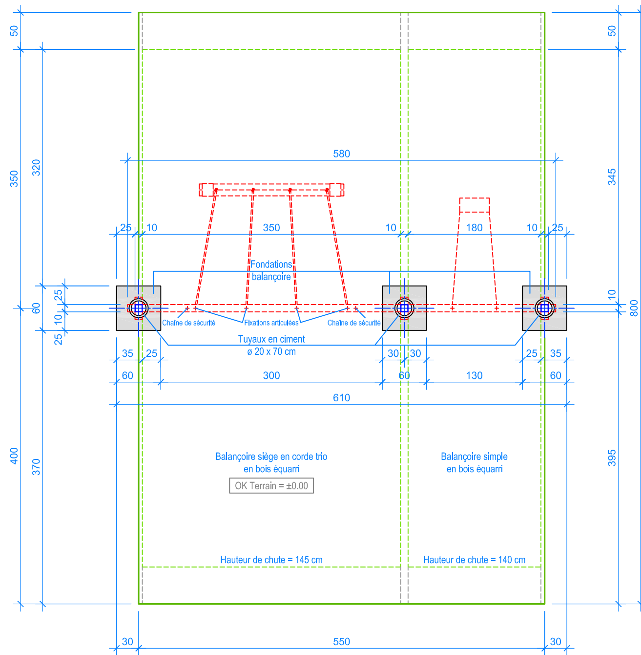
PLAN 1:50
