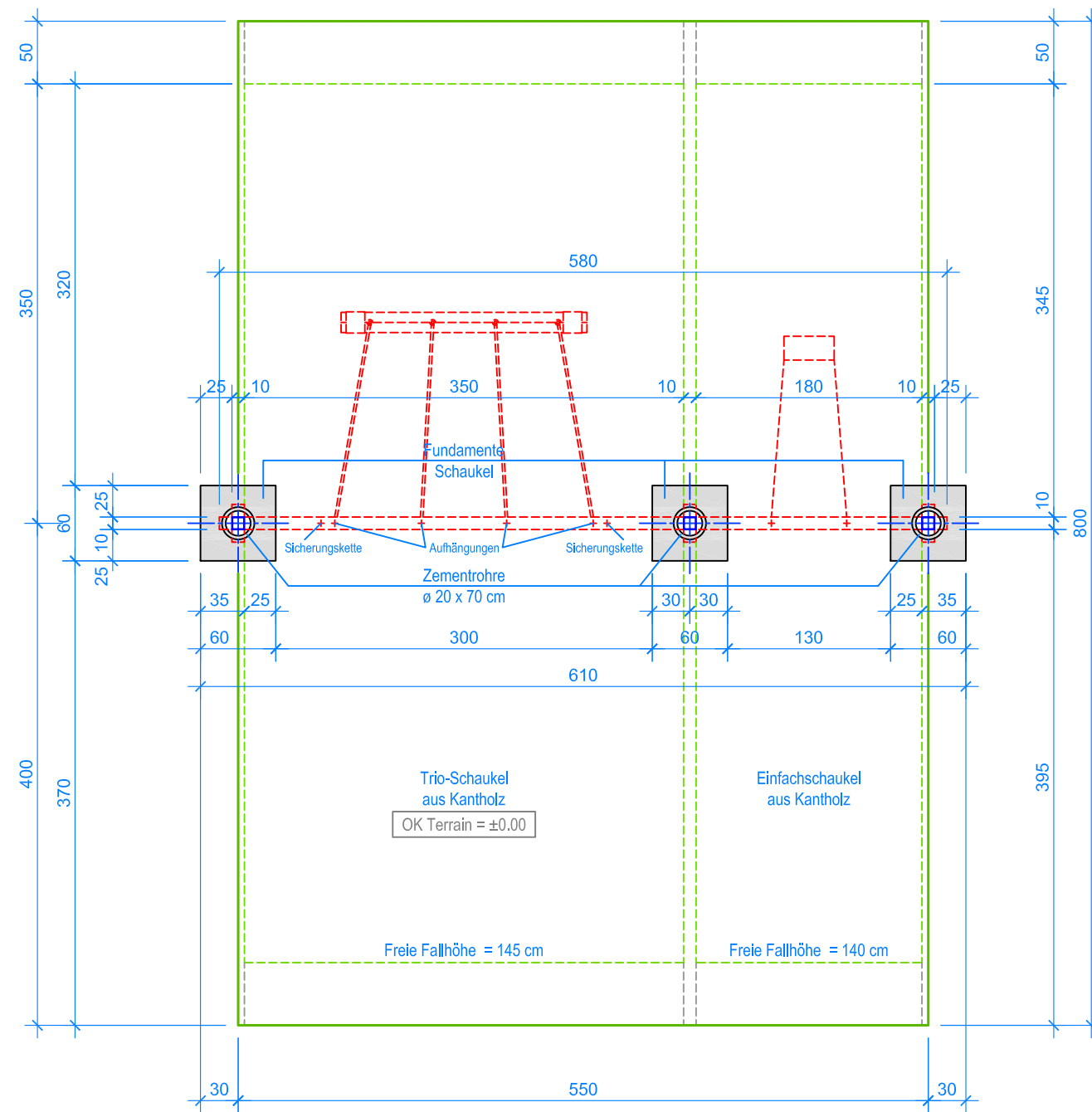
GRUNDRISS 1:50
