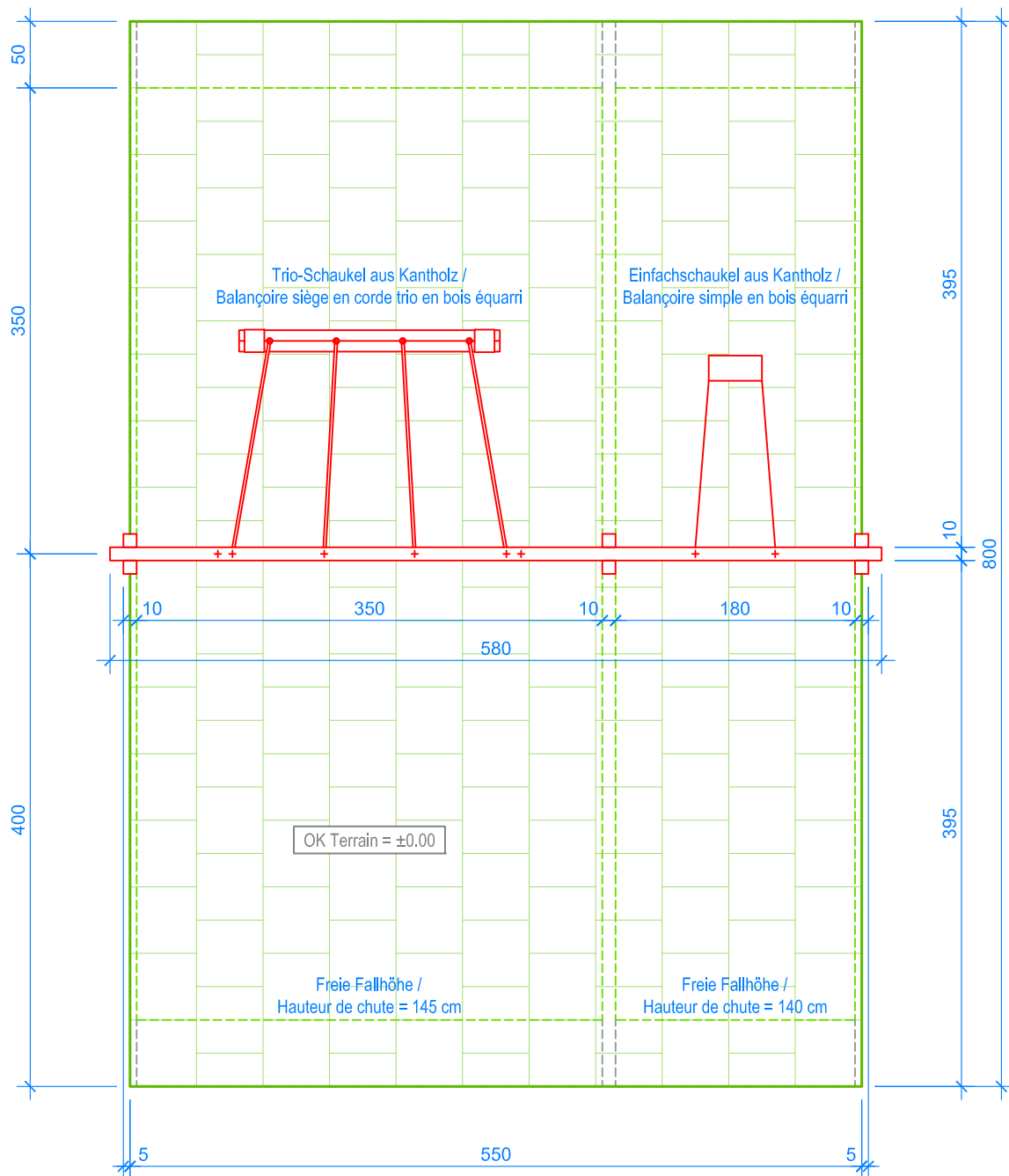
GRUNDRISS / PLAN 1:50
