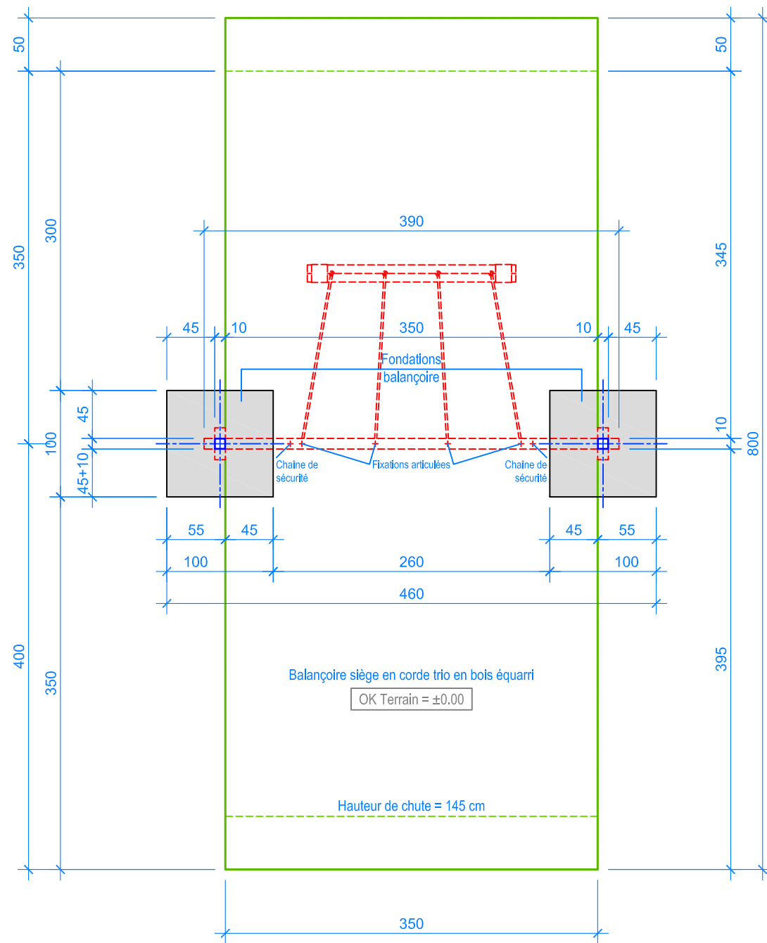
PLAN 1:50
