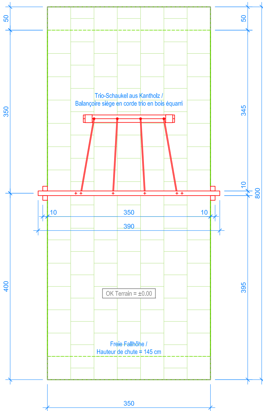
GRUNDRISS / PLAN 1:50
