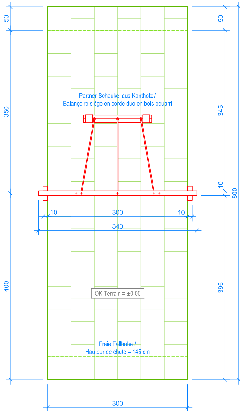
GRUNDRISS / PLAN 1:50
