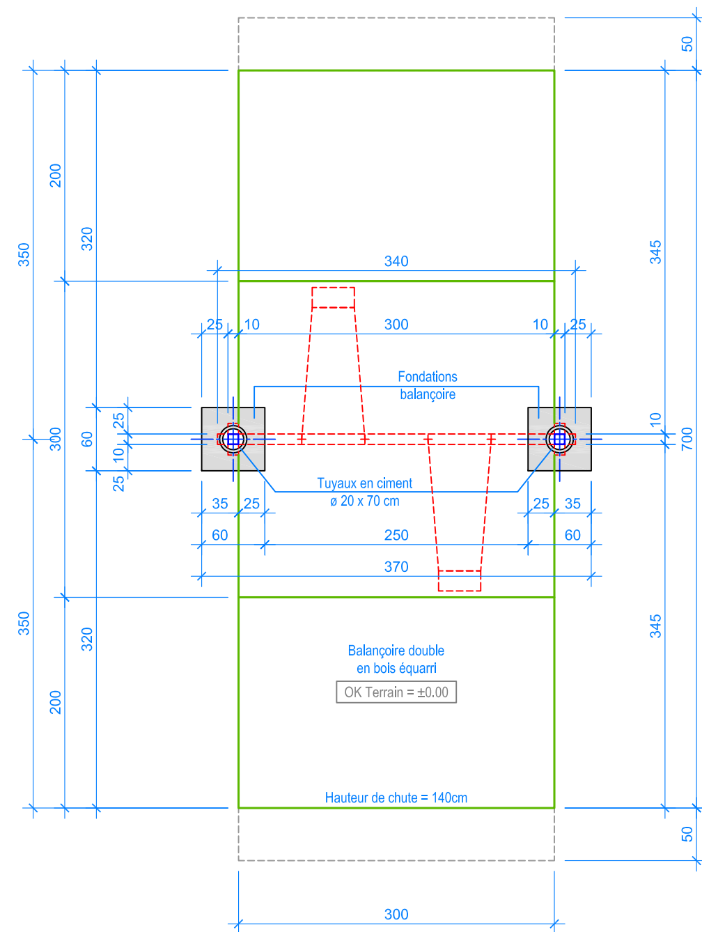
PLAN 1:50
