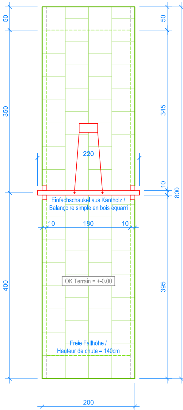
GRUNDRISS / PLAN 1:50
