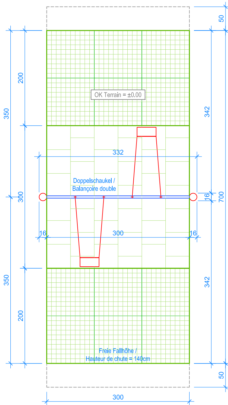
GRUNDRISS / PLAN 1:50
