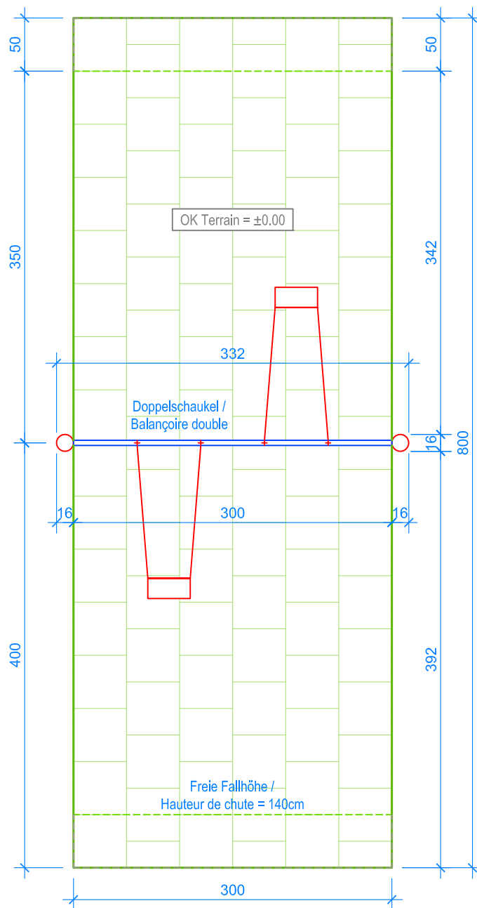
GRUNDRISS / PLAN 1:50
