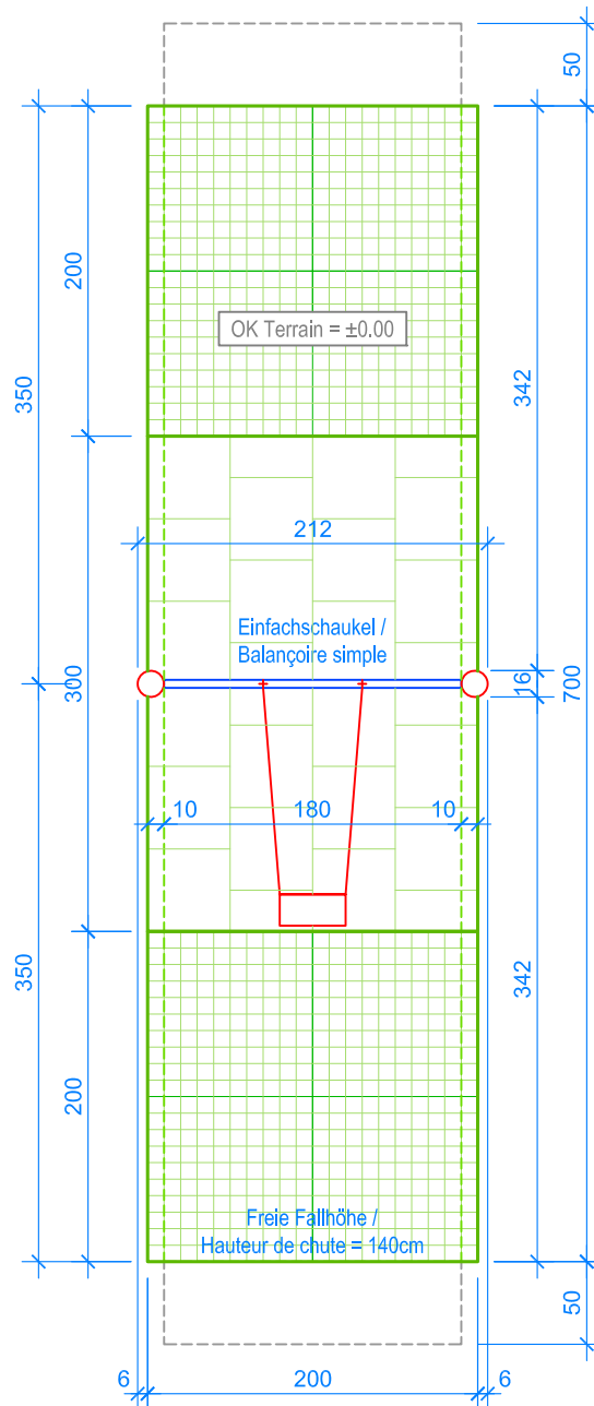
GRUNDRISS / PLAN 1:50
