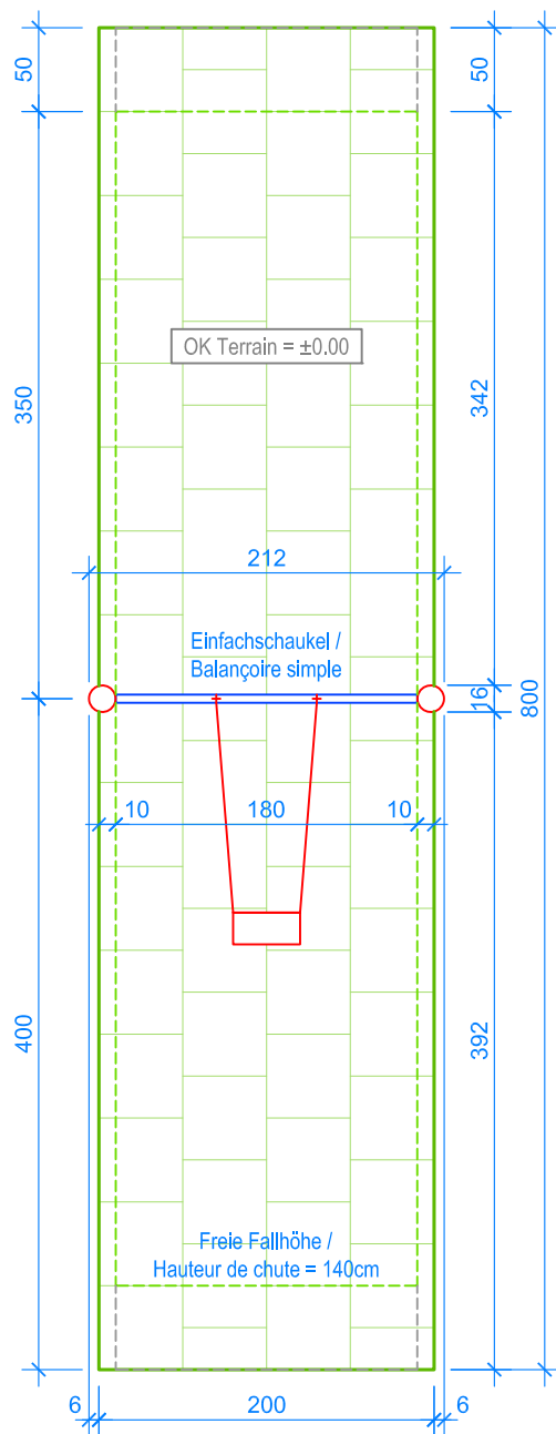
GRUNDRISS / PLAN 1:50
