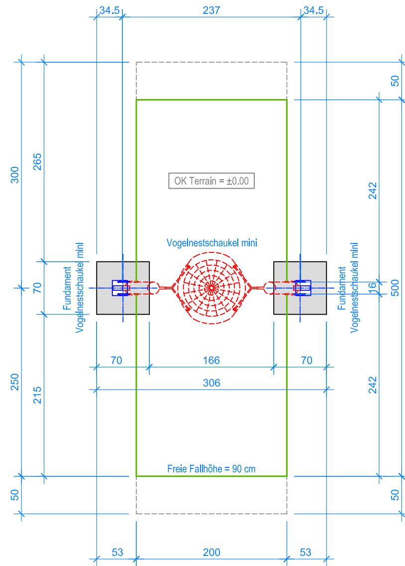
GRUNDRISS 1:50
