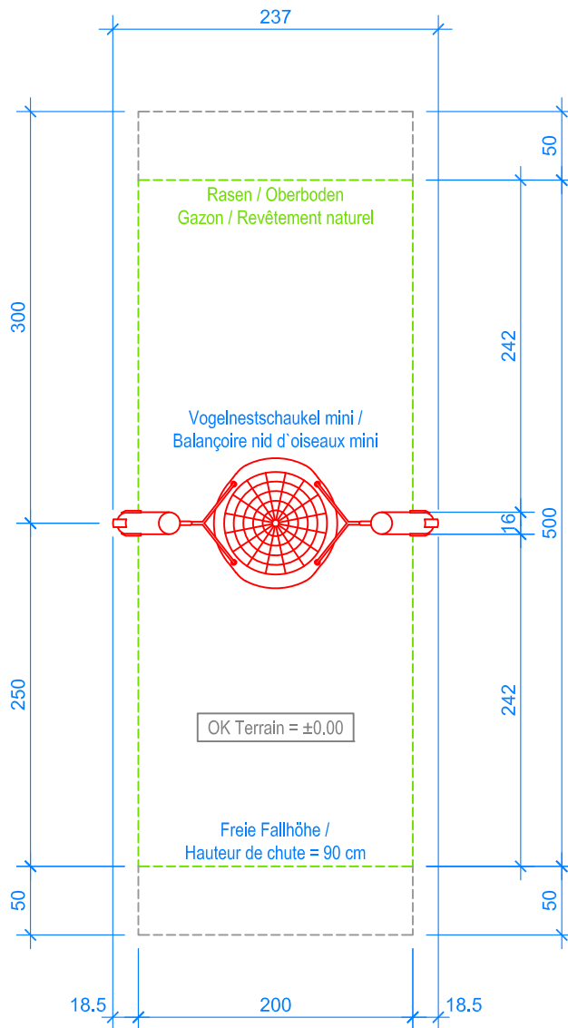
GRUNDRISS / PLAN 1:50
