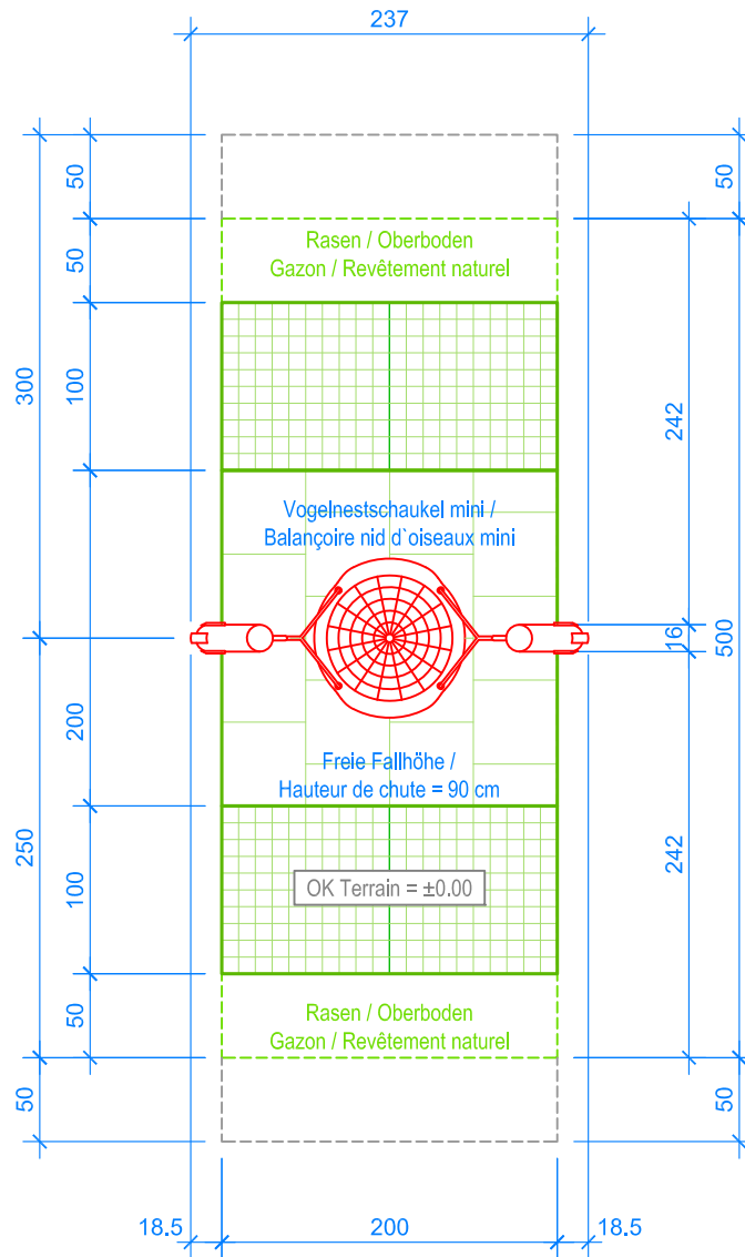
GRUNDRISS / PLAN 1:50
